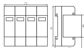
KSD-T2 275/160 3P+N
